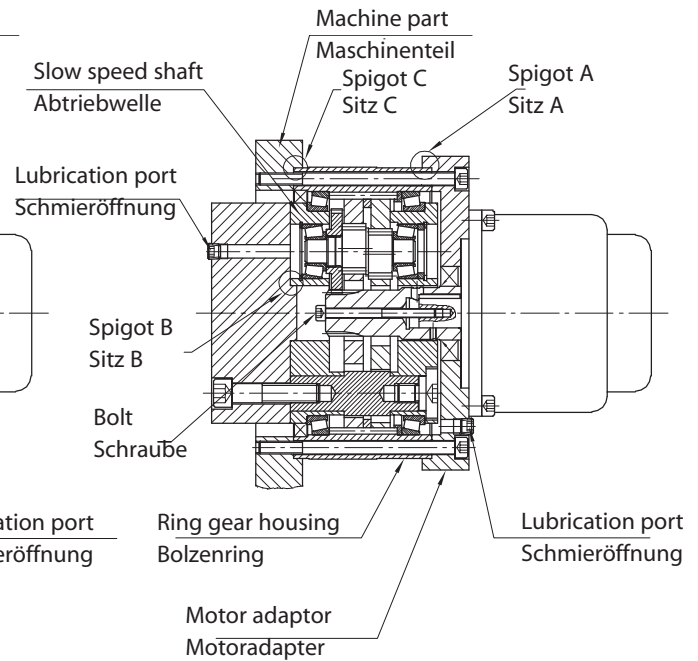
Abb. 32b Einbautoleranzen
